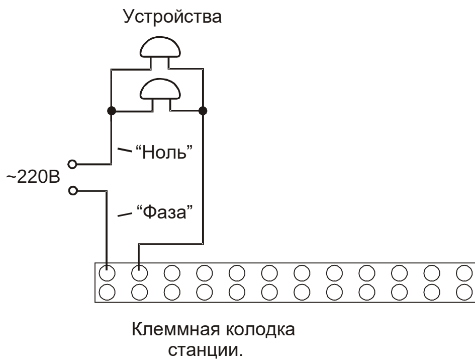
Рис. 2 Схема для второго канала (второго реле)
